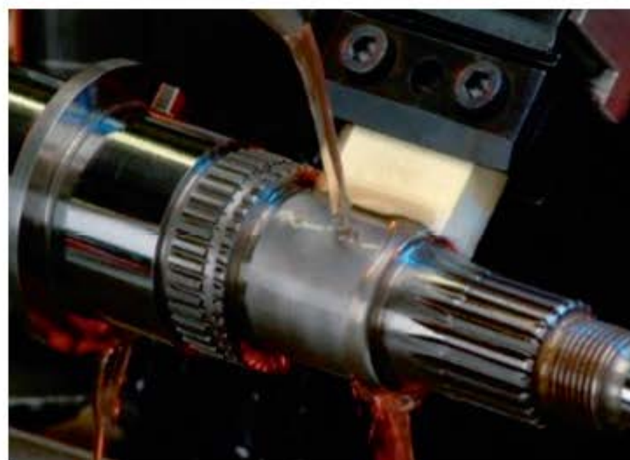
Getriebewelle zwischen Spitzen auf der Steinfinishmaschine. Bild: Nagel
